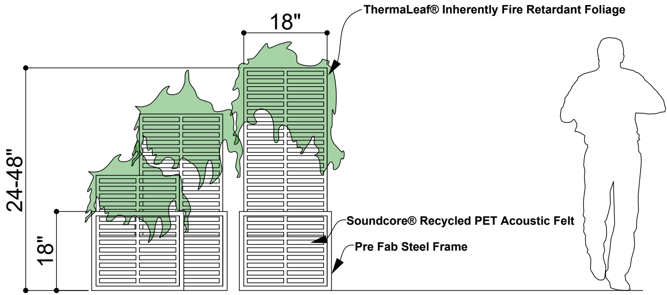
① ELEVATION 1
